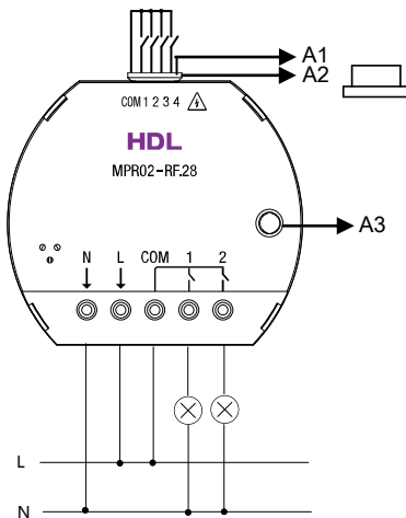
Figure 4. Wiring 图 4. 接线图
